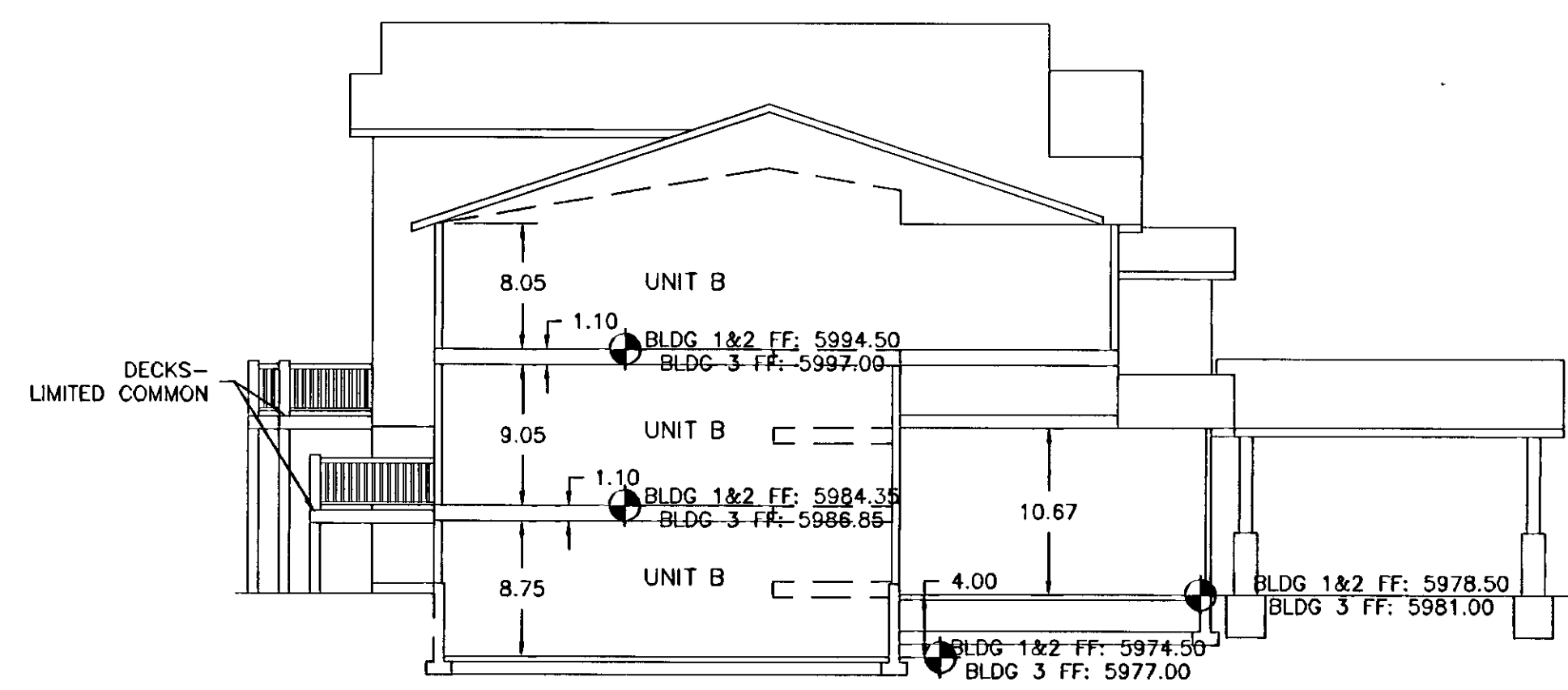
SECTION B-B SCALE: 1"=10'
