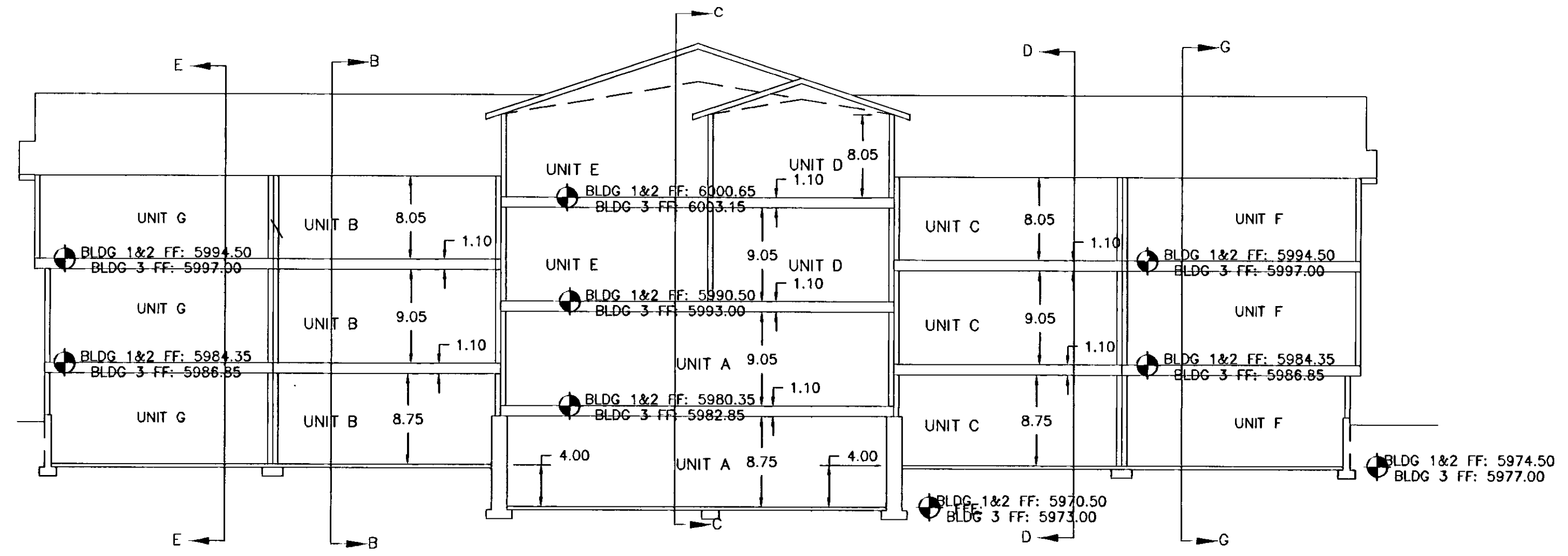
SECTION A-A SCALE: 1"=10'
