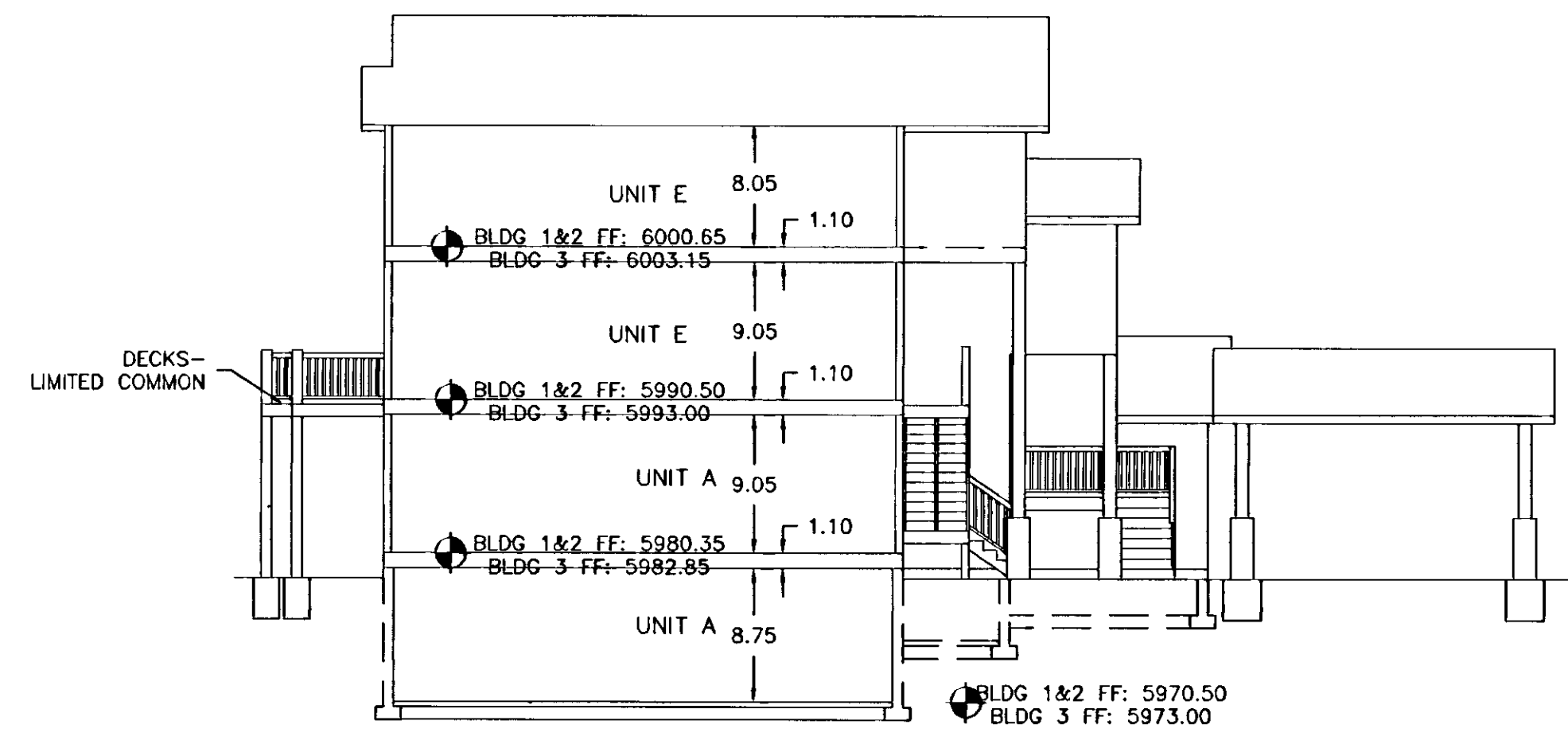
SECTION C-C SCALE: 1"=10'
