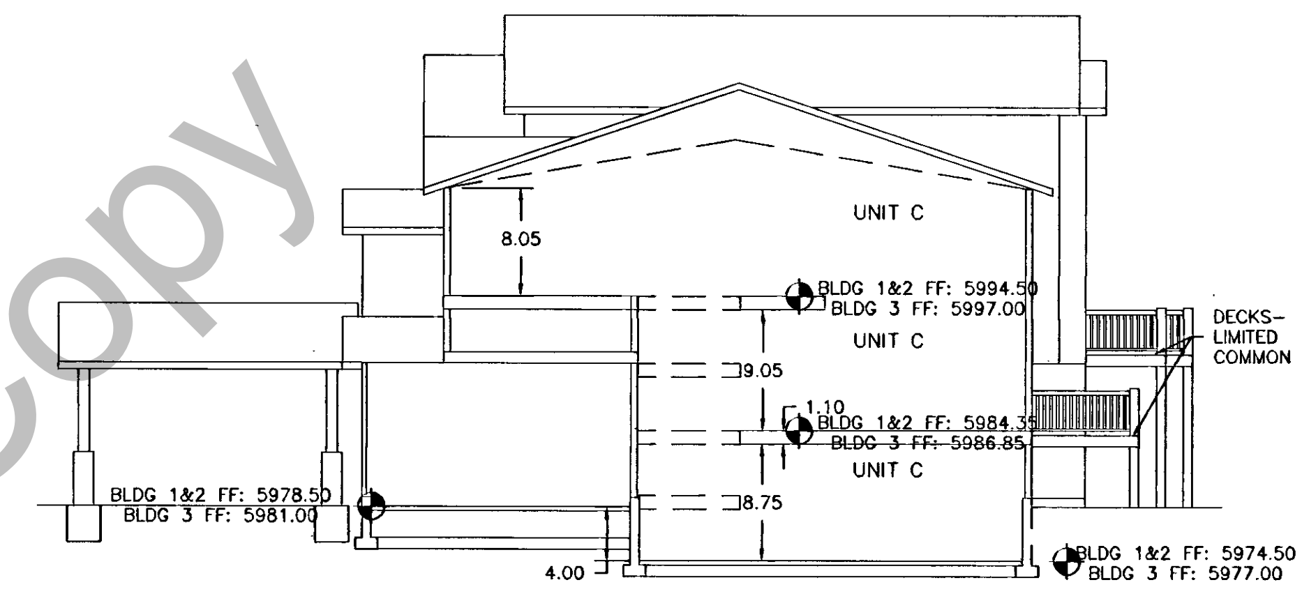
SECTION D-D SCALE: 1"=10'
