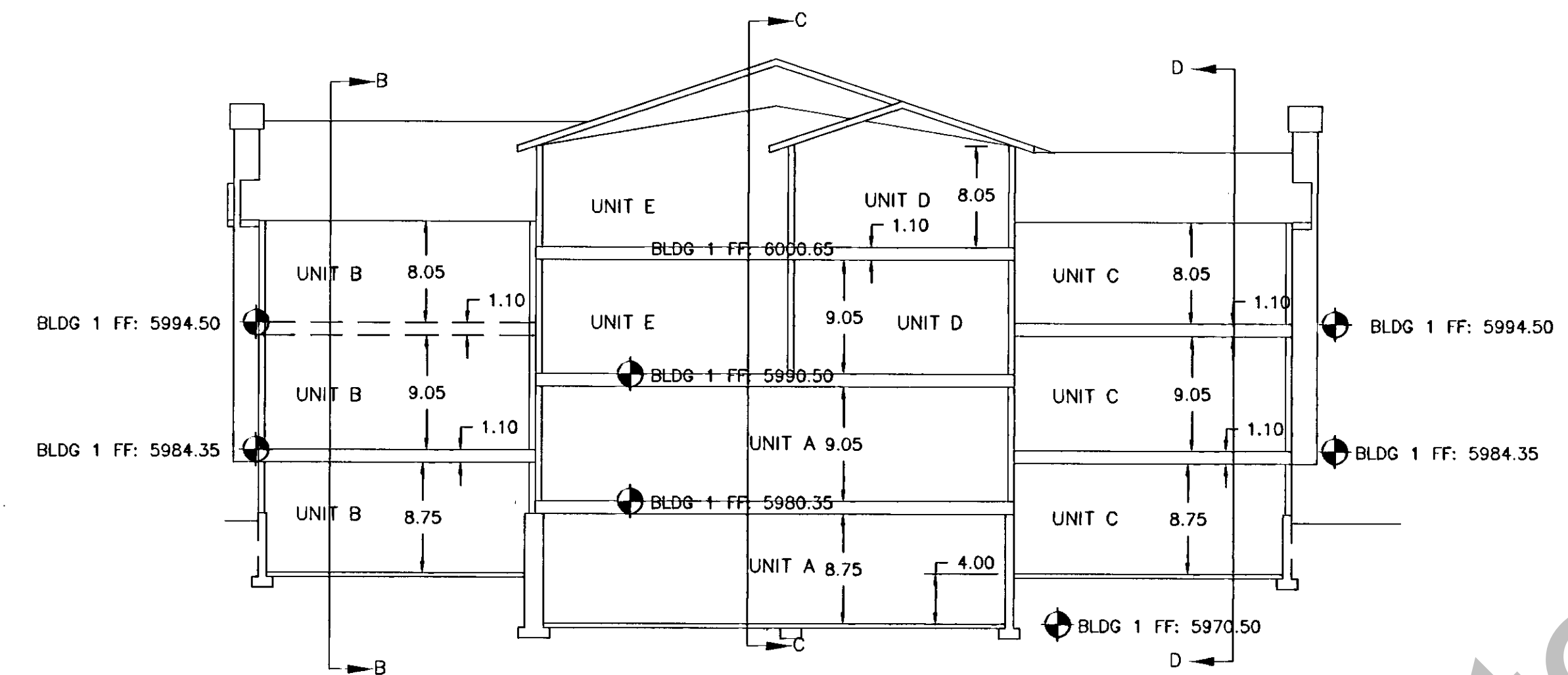
SECTION A2-A2 SCALE: 1"=10'
