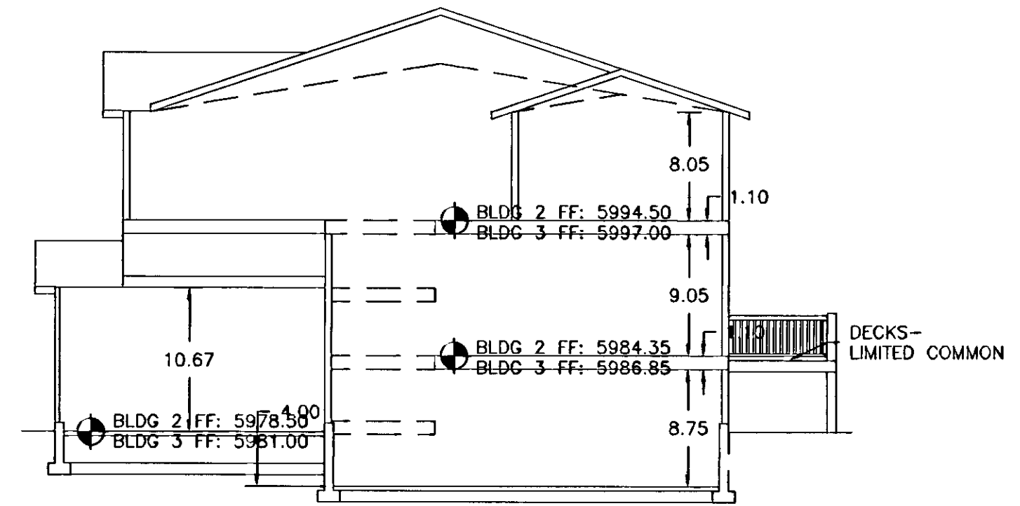
SECTION G-G SCALE: 1"=10'
