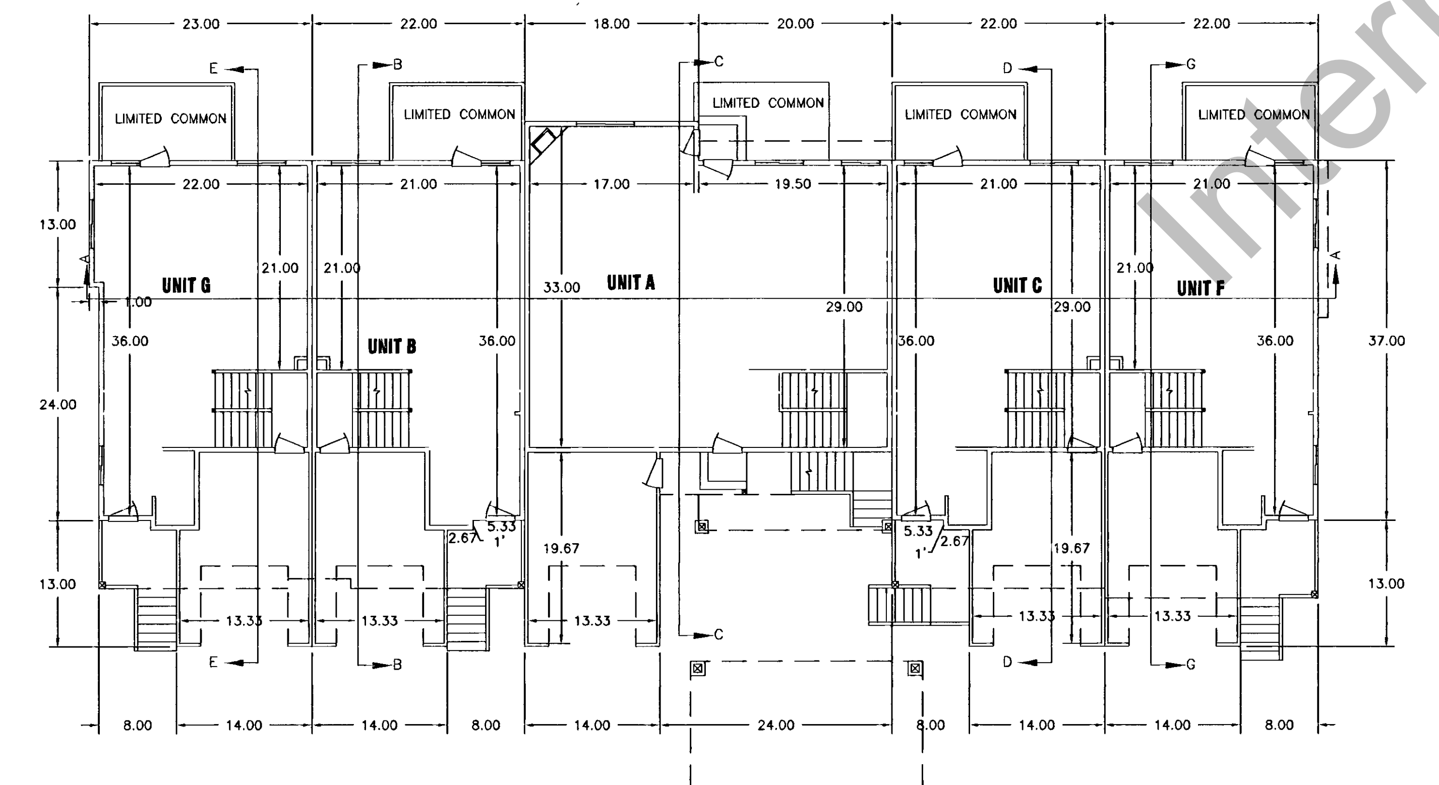
MAIN LEVEL SCALE: 1"=10'
