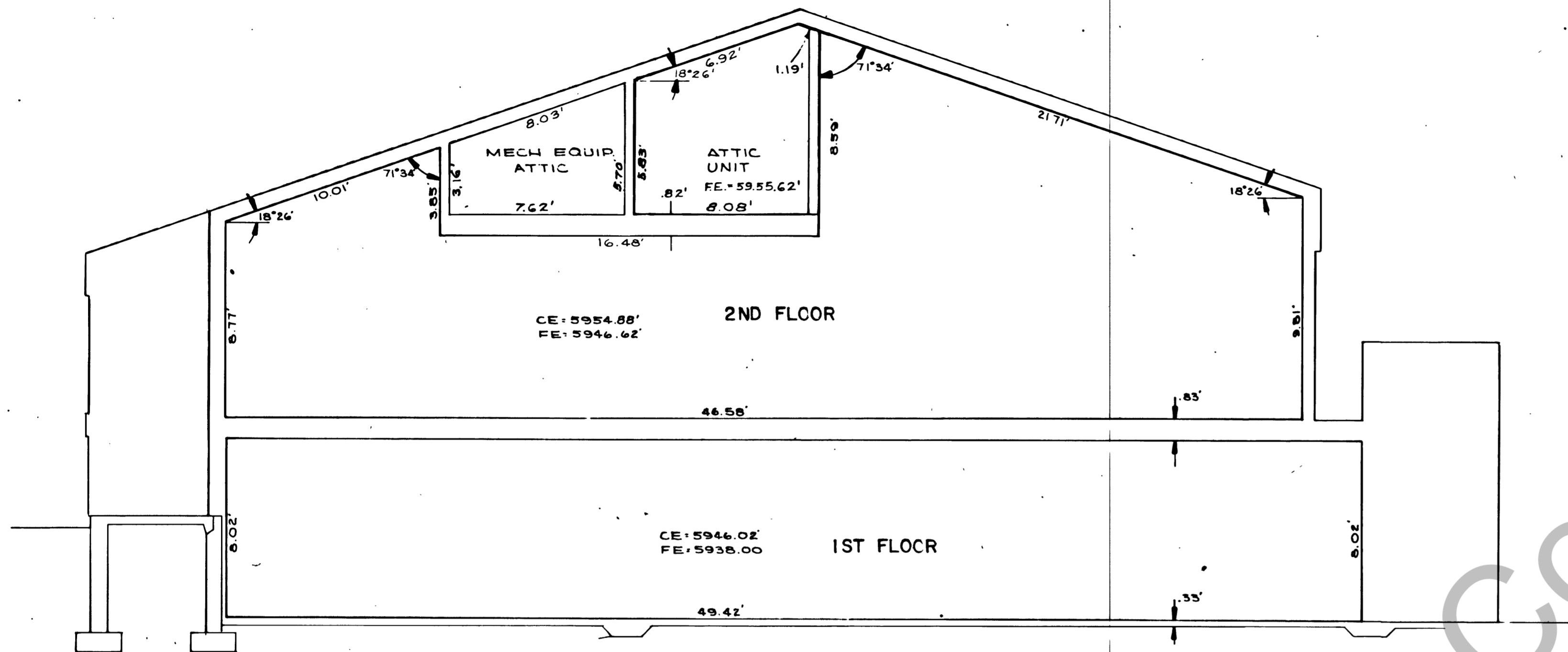
B SECTION SCALE: 1" = 4'
