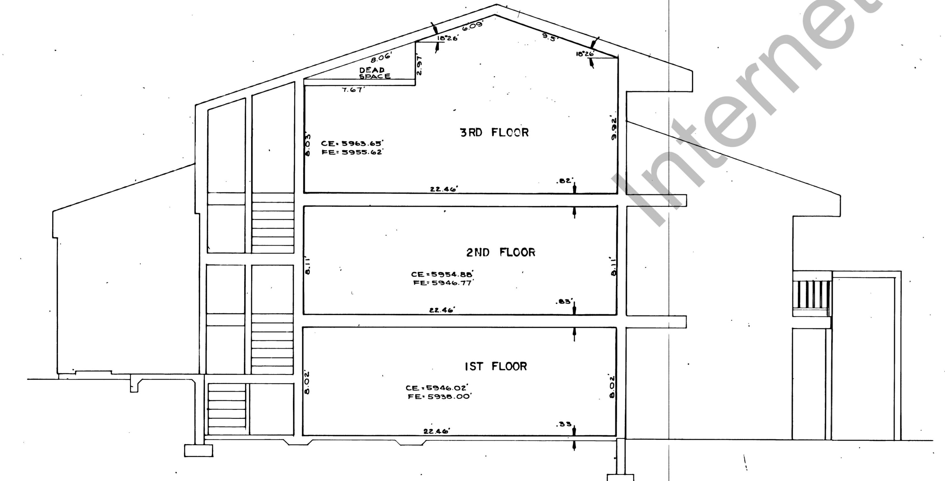
A SECTION SCALE: 1" = 4'
