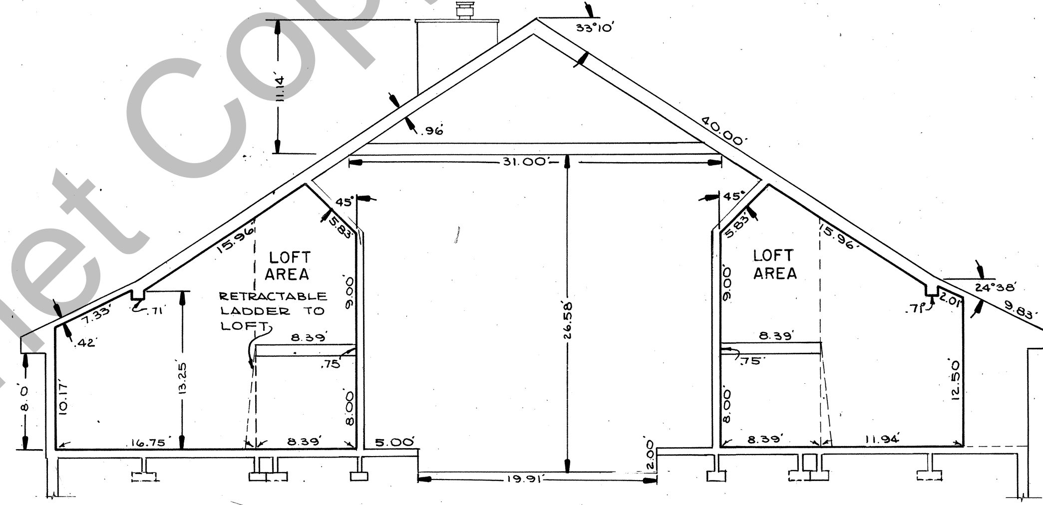
SECTION A-3 SCALE: 1" = 8"
